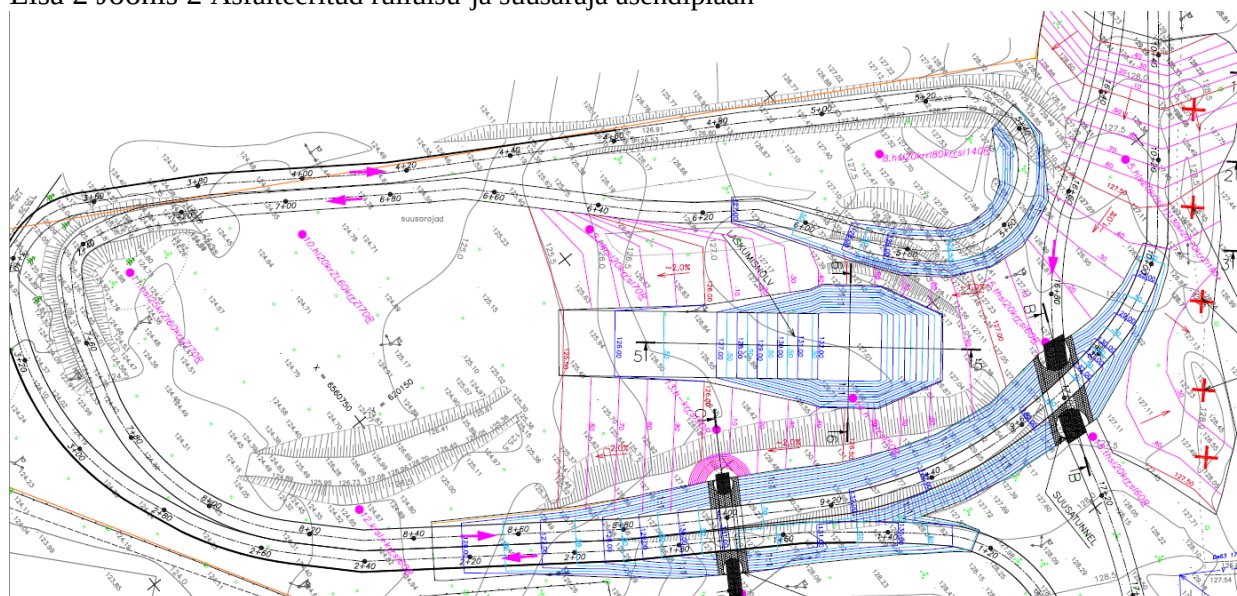
Lisa 2 Joonis 2 Asfalteeritud rulluisu-ja suusaraja asendiplaan
